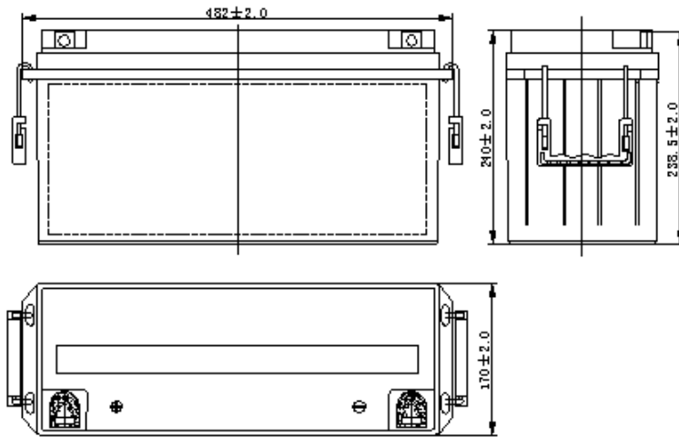
外形尺寸图
