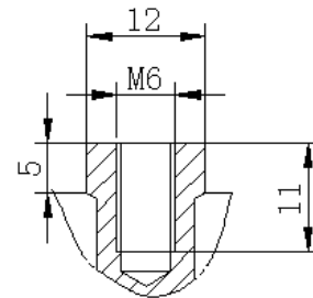
端子尺寸图
