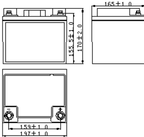
外形尺寸图
